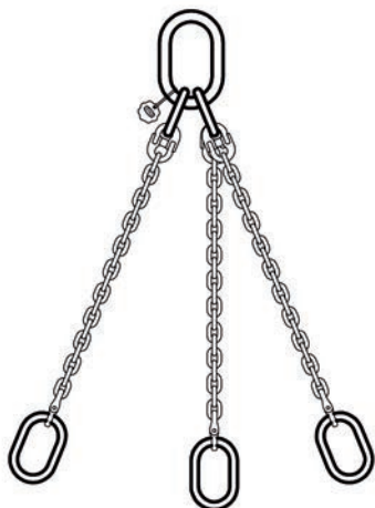
TIPO A3 ANILLA + 3 CADENAS + 3 ANILLAS
